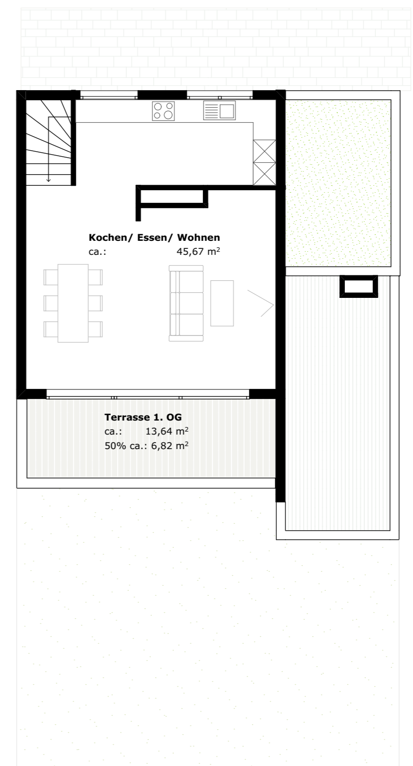
Grundriss 1. Obergeschoss
