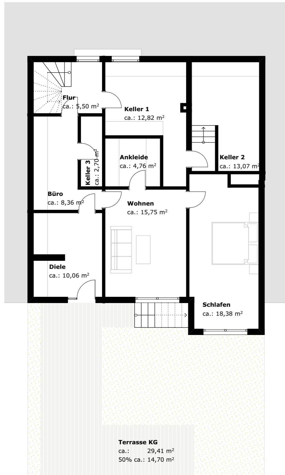
Grundriss Kellergeschoss
